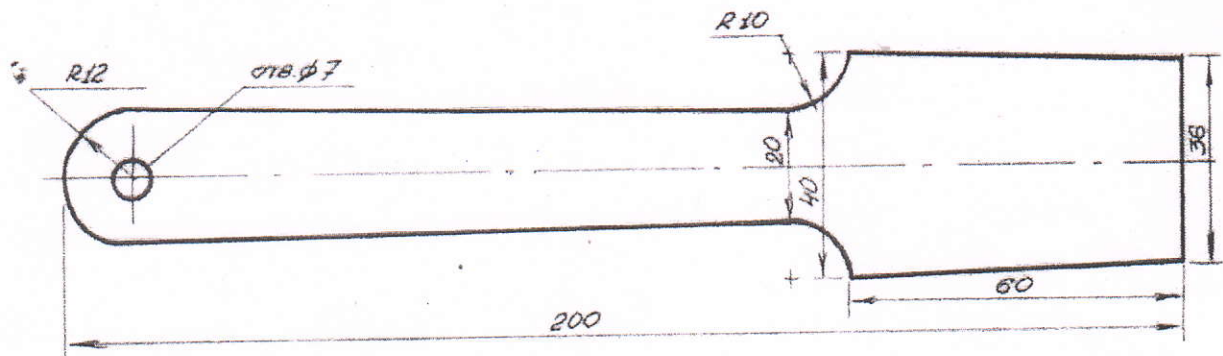
Рис. 1. Лопатка кухонная
